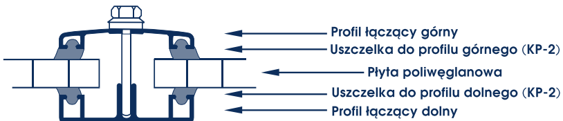
łączenie przy pomocy profili aluminiowych
